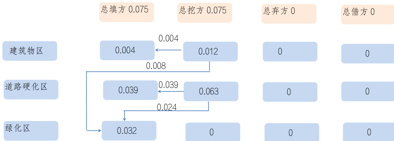
图 1-2 土石方平衡流向图 单位：万 \text{m}^3
